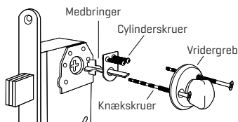
Indvendig side
